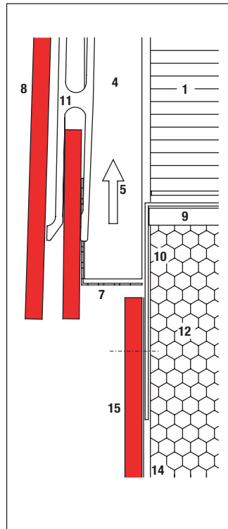
Holz/Metall-Unterkonstruktion
