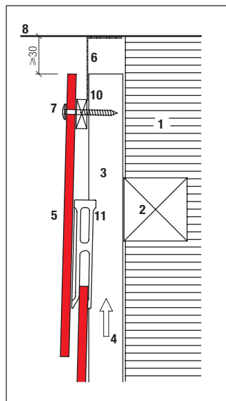
Anschluss an Dachuntersicht
