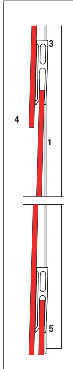
Prinzipieller Schnitt Fassadenfuß
