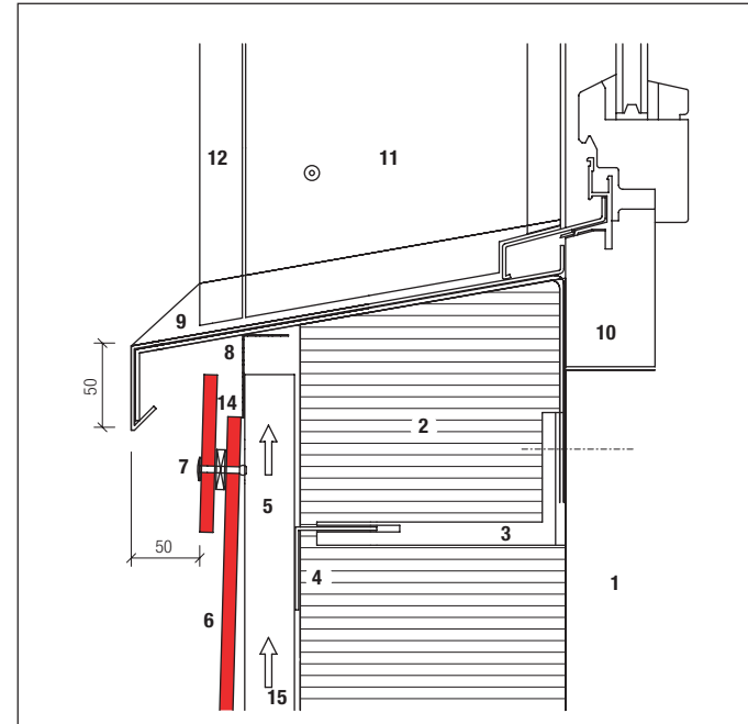
Metallfensterbank
