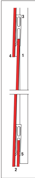
Prinzipanschnitt Fassadenfuss
