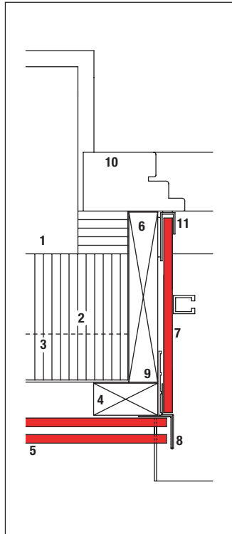
SWISSPEARL-Leibung
