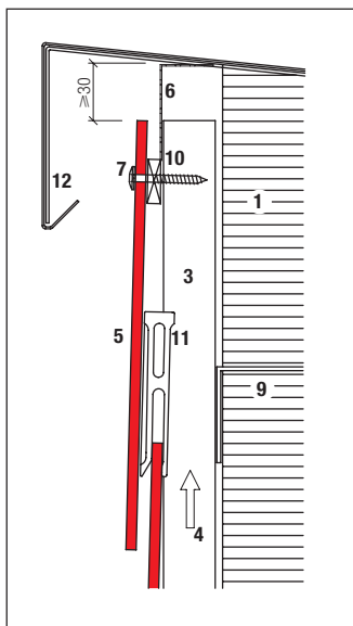
Dachrandabschluss
