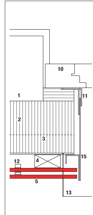
Steckzarge
