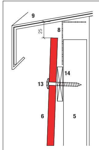
Fensterbankanschluss
