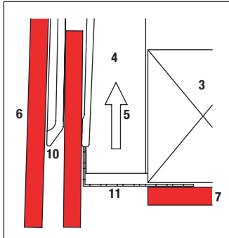
Fassadenplatte überstehend
