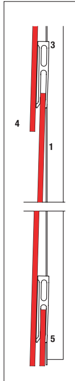
Prinzipialschnitt Fassadenfuß
